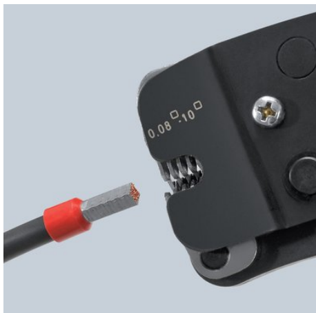
Négyszög-krimp
